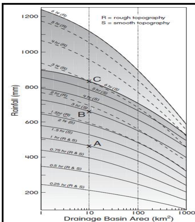
شکل ۶-۶- حداکثر بارش محتمل بر مبنای زمان در وسعت حوضه زهکشی (اداره هواشناسی استرالیا، ۱۹۸۴).
