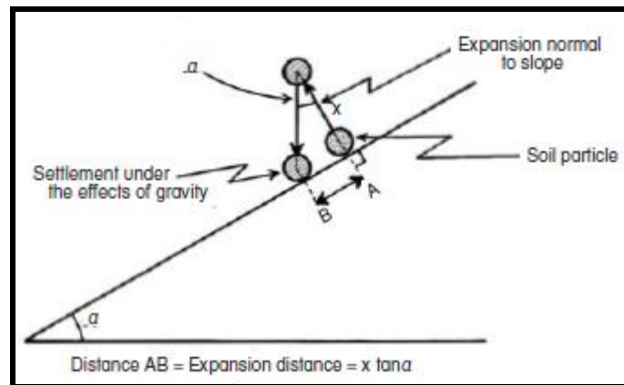
شکل ۱۲-۹- مکانیزم جابه‌جایی رو به پایین مواد در سراشیبی در اثر خزش خاک.
