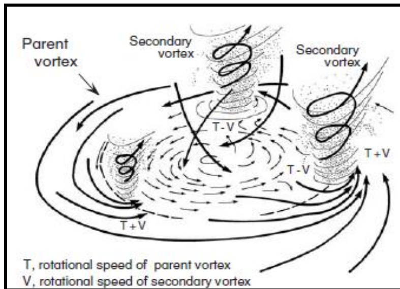
شکل ۴-۱۱- مدل شکل‌گیری چرخندگی چندگانه در یک تورنادو (بر اساس فوجیتا، ۱۹۷۱ و گرازبولیس، ۱۹۹۳).
