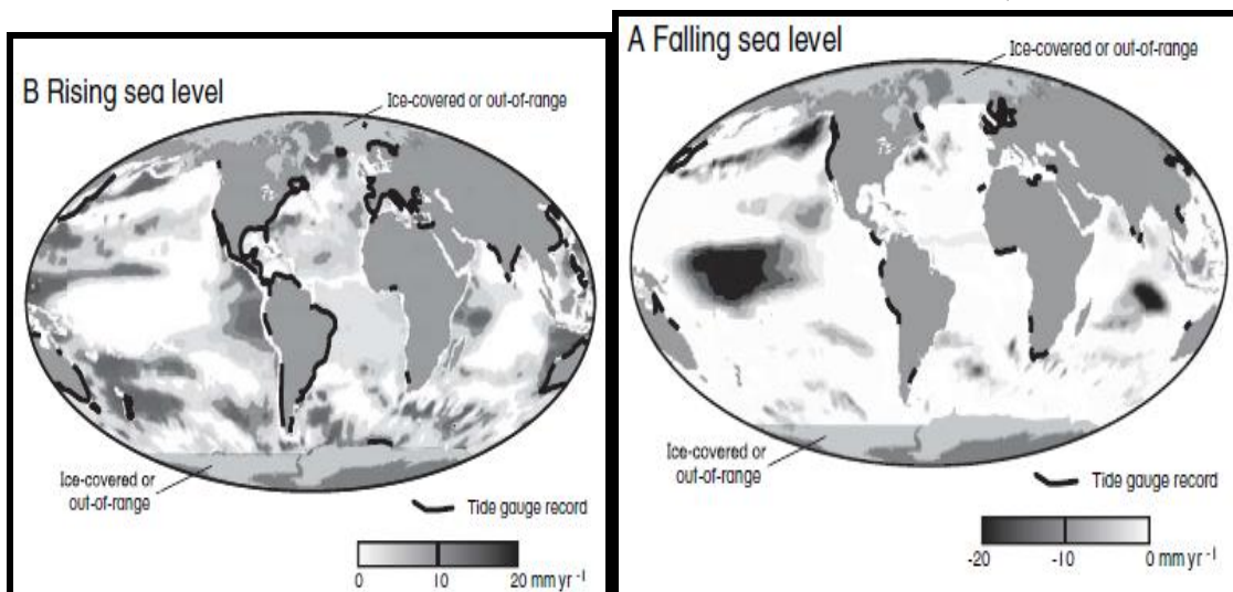
شکل ۸-۱۰- تغییرات جهانی سطح دریا بر اساس داده‌های جزر و مد سنج‌های ساحلی در بین سال‌های ۱۹۶۰ و ۱۹۷۹ (از برایانت، ۱۹۸۸) و داده‌های ارتفاع سنج ماهواره TOPEX/POSEIDON بین ژانویه ۱۹۹۳ و دسامبر ۱۹۹۹ (A). کاهش‌ها (B) افزایش‌ها (کازینو، ۲۰۰۲).
