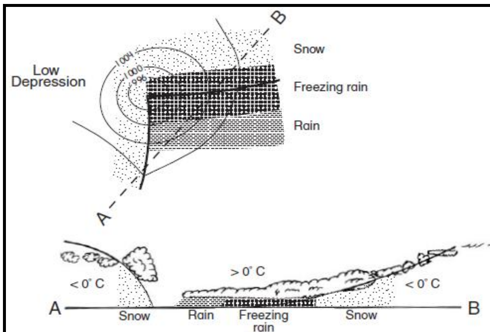
شکل ۳-۲۰- نمایش شماتیک از الگوهای بارش یک کم‌فشار سیکلونی عرض‌های میانه در فصل زمستان در نیمکره شمالی.
