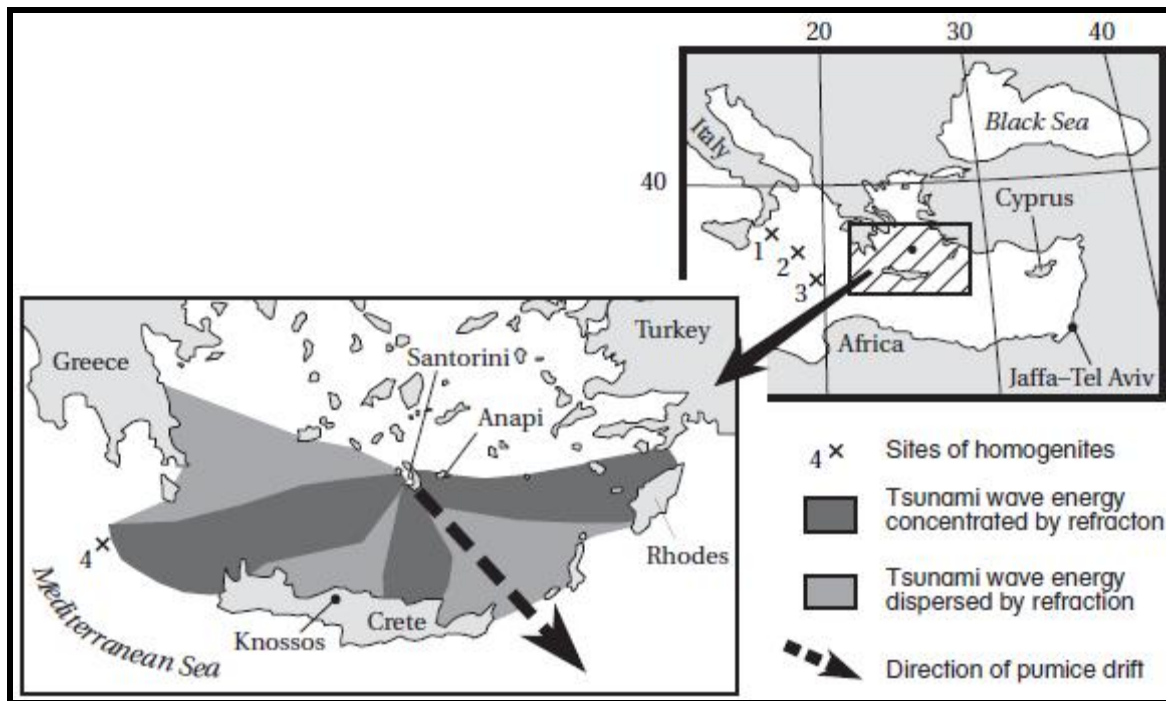
شکل ۱۱-۶- منطقه مدیترانه شرقی که به دلیل فوران سانترونی در حدود سال ۱۴۷۰ قبل از میلاد تحت تاثیر قرار گرفت. اعداد سایت‌های دارای ویژگی‌های یکسان را نشان می‌دهند: (۱) پشته کالبرین (۲) دشت مگاکی دریای یونان (۳) حوضه بن ناک (۴) پشته مدیترانه. الگوهای پراکنش بر اساس کاستنز و سیتا (۱۹۸۱).
