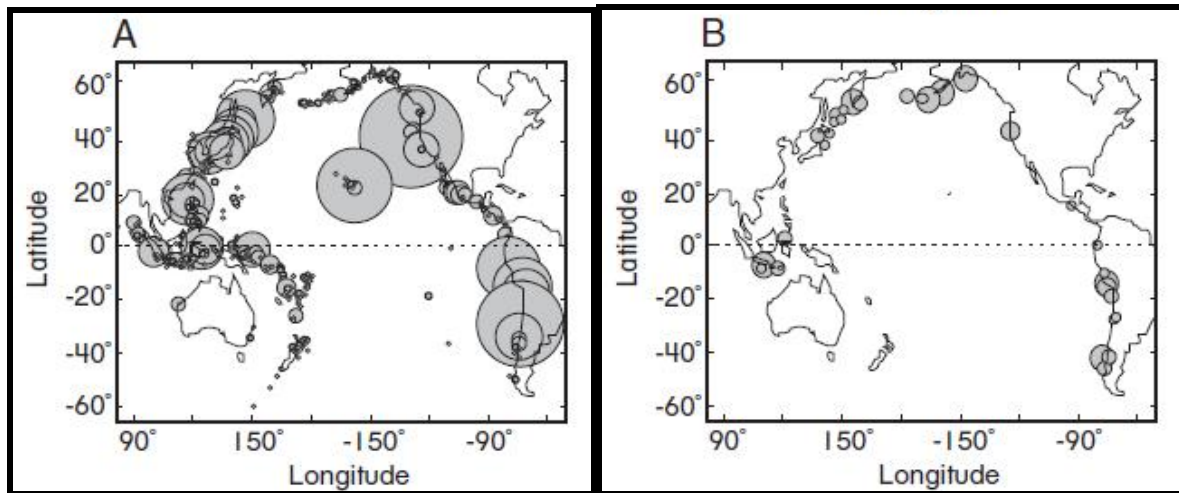
شکل ۱۰-۱۱- A) توزیع فضایی سونامی‌ها از ۴۷ سال قبل از میلاد؛ B) مناطق منشاء برای حوادث اقیانوس آرام (اقتباس از داده‌های مرکز ملی ژئوفیزیک و مرکز جهانی داده‌های ژئوفیزیک زمین جامد، ۱۹۸۴).
