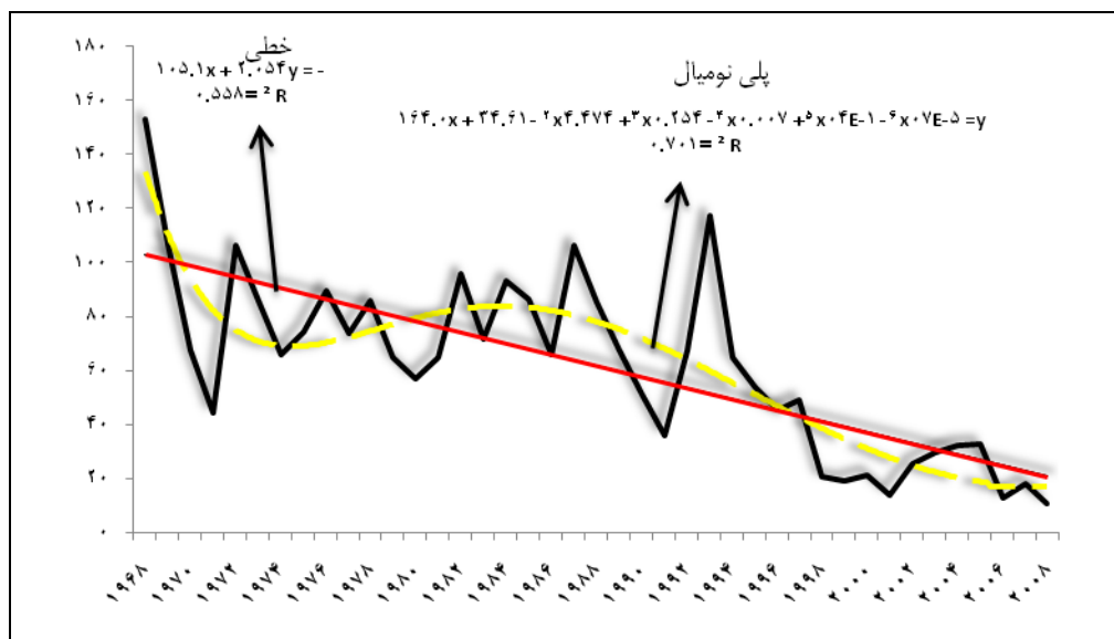
شکل ۸. تغییرات سری زمانی فصل زمستان دبی حوضه ارس طی بازه زمانی چهل ساله
